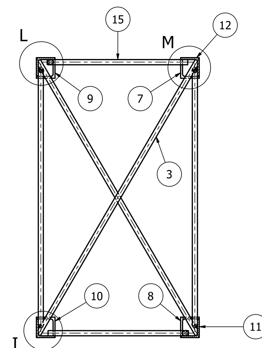
SNITT D-D ( 1:10 )
