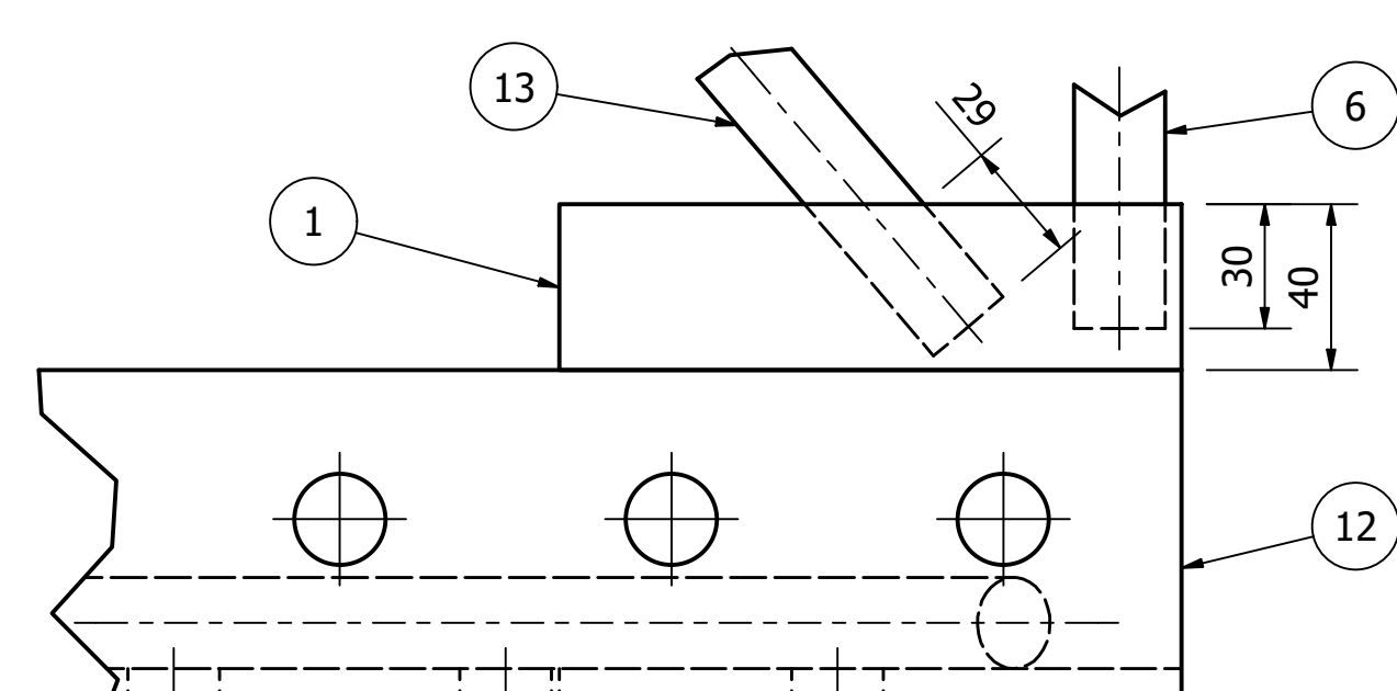
G(1:2)
