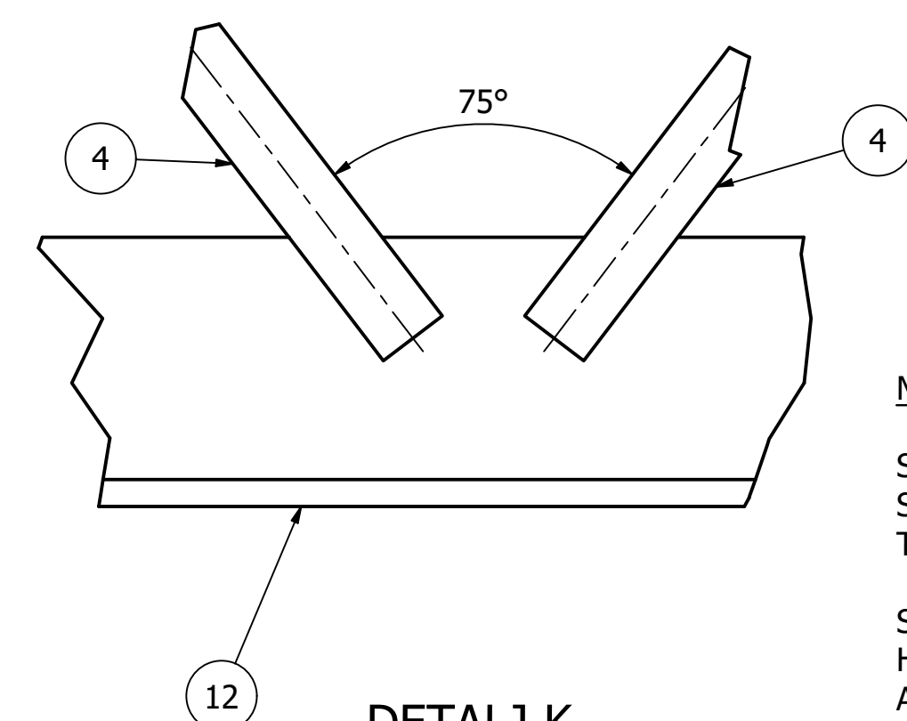
DETALJ K ( 1 : 2 )
