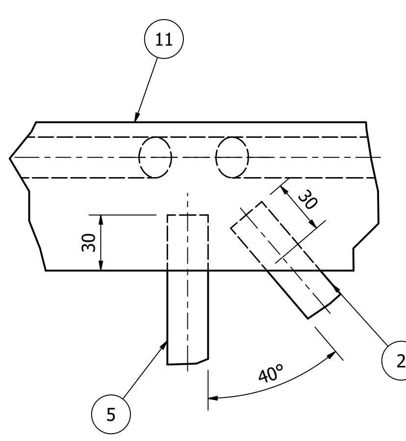
DETALJ J ( 1 : 2 )
