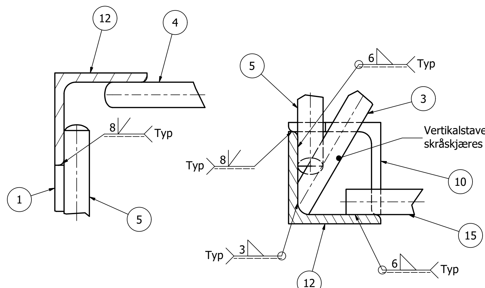
DETALJ H ( 1 : 2 )
